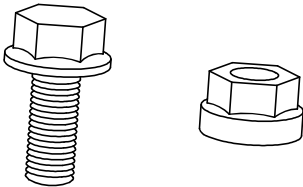
24X M8X20
