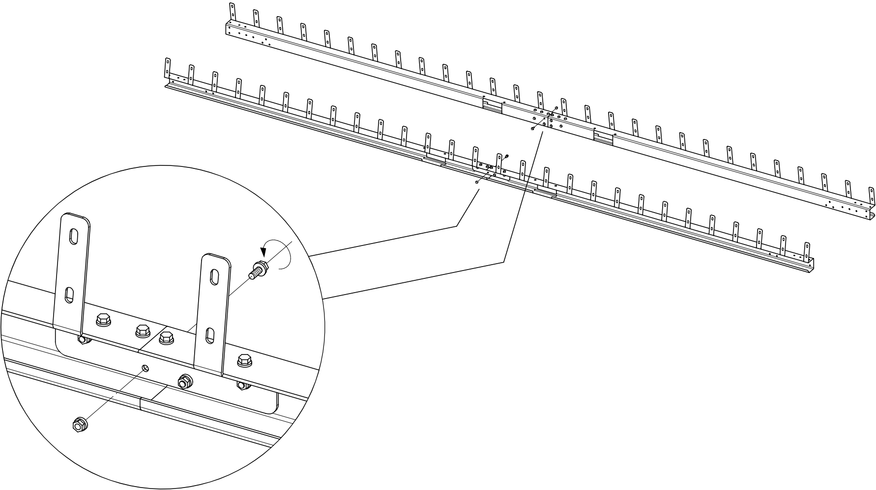
24X M8X20
